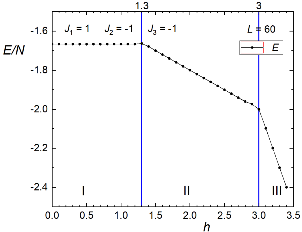
Рис. 2.5. Полевая зависимость энергии основного состояния системы E .
