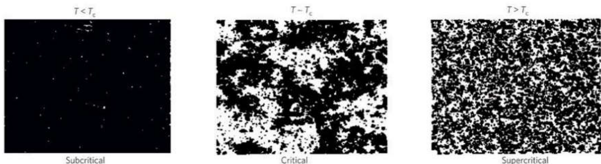
Рис. 1.1. Модели Изинга при различных температурах.
